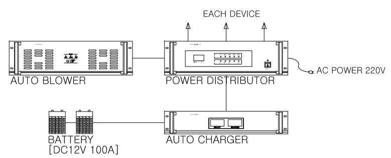
IBS5250-PA08N 계통도 SCALE : 1/NONE (A3)
