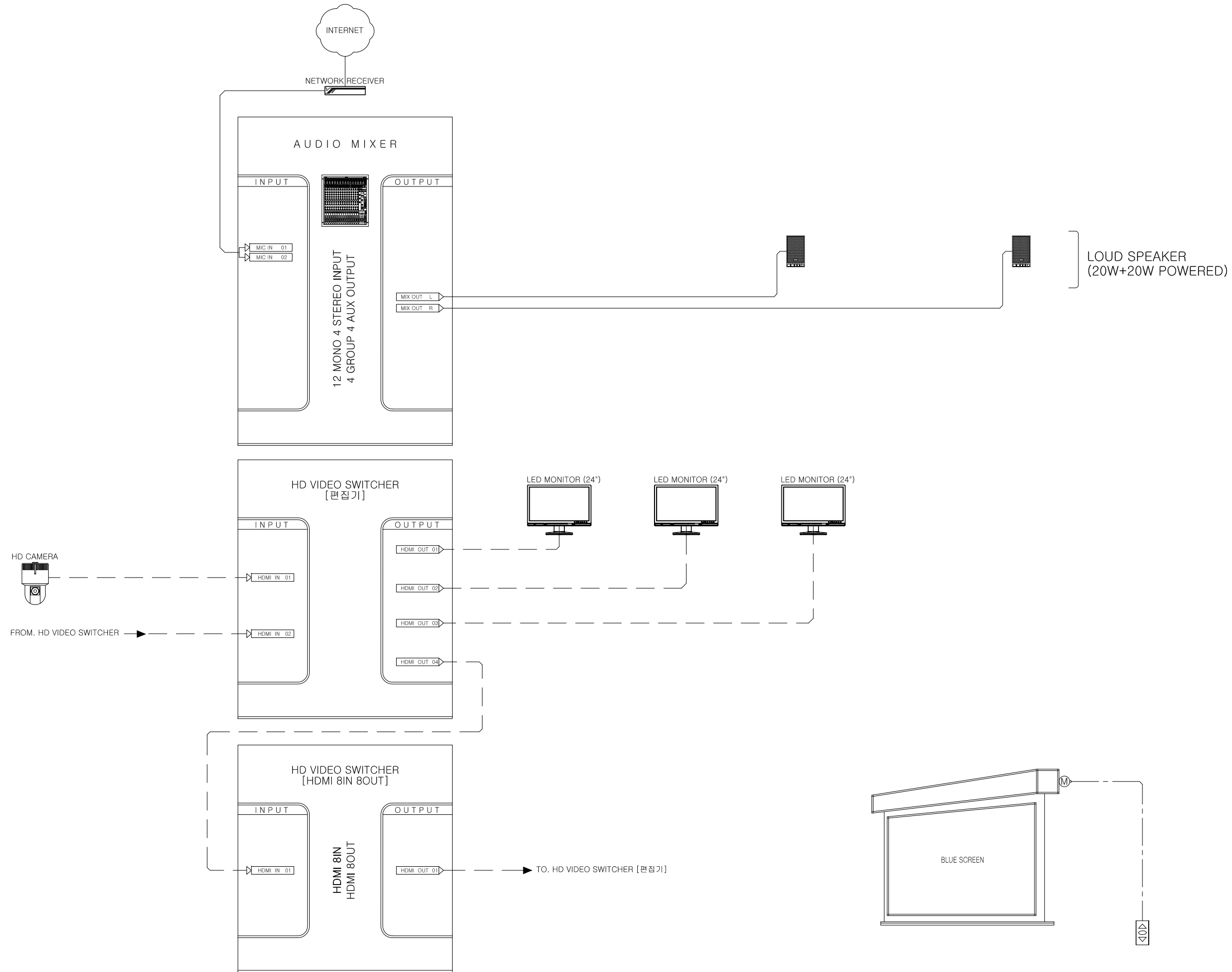
IBS5250-V02N 계통도 SCALE : 1/NONE (A3)
