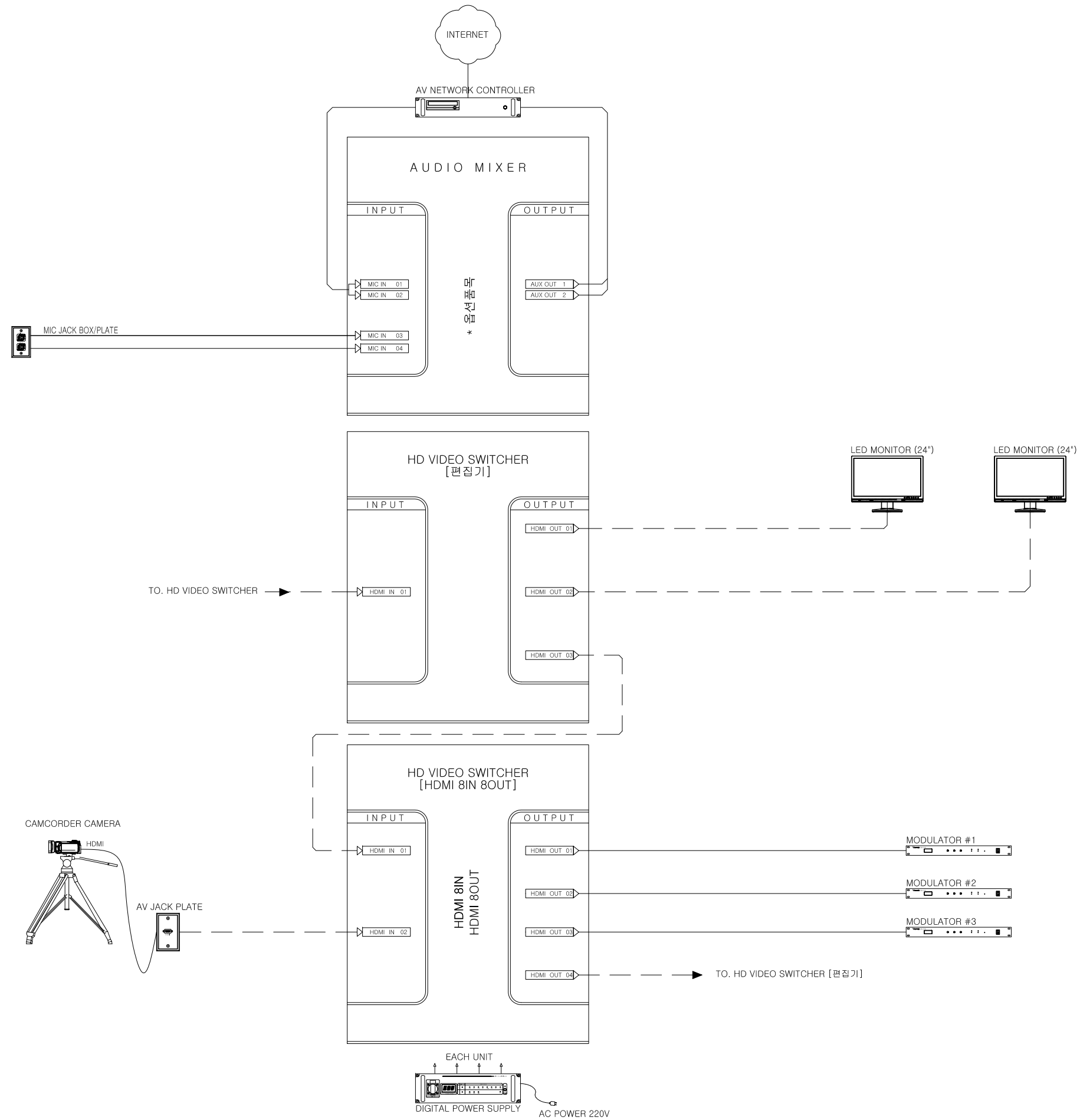
IBS5250-V09 계통도 SCALE : 1/NONE (A3)
