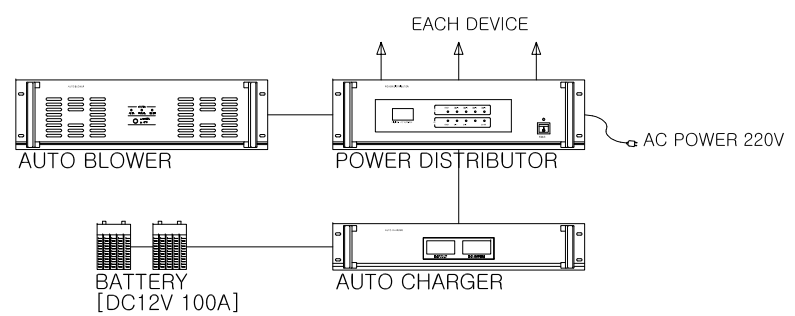
IBS5250-PA08 계통도 SCALE : 1/NONE (A3)
