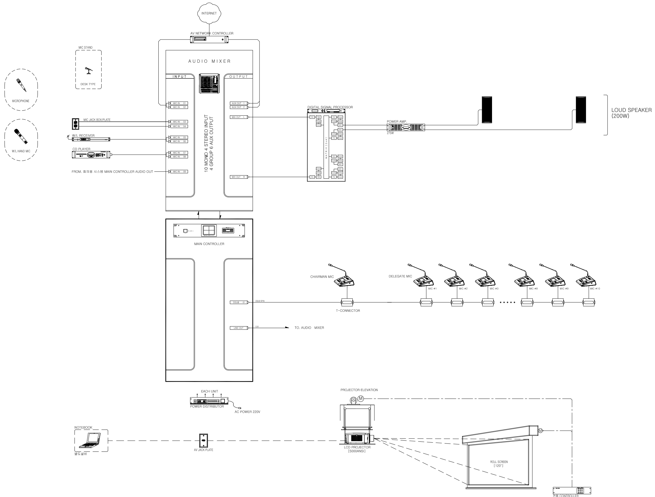
IBS5250-CR05 계통도 SCALE : 1/NONE (A3)
