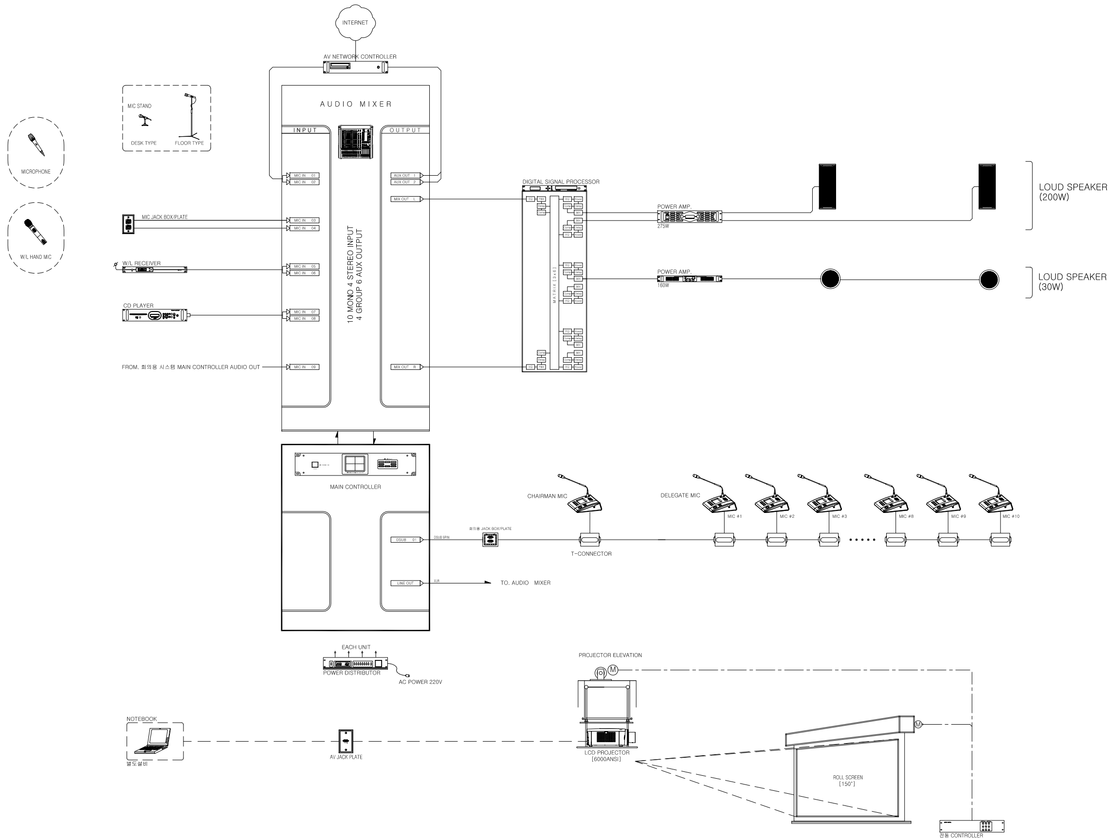
IBS5250-CR06 계통도 SCALE : 1/NONE (A3)
