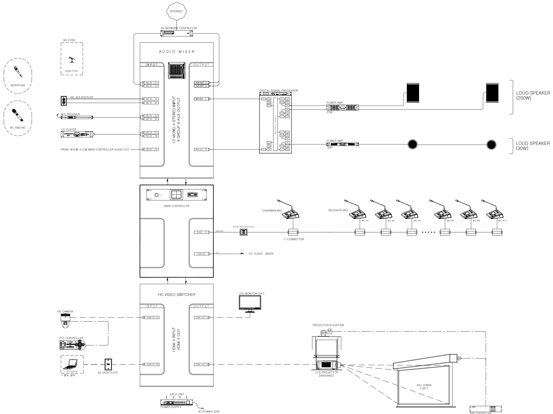
IBS5250-CR08 계통도 SCALE : 1/NONE (A3)
