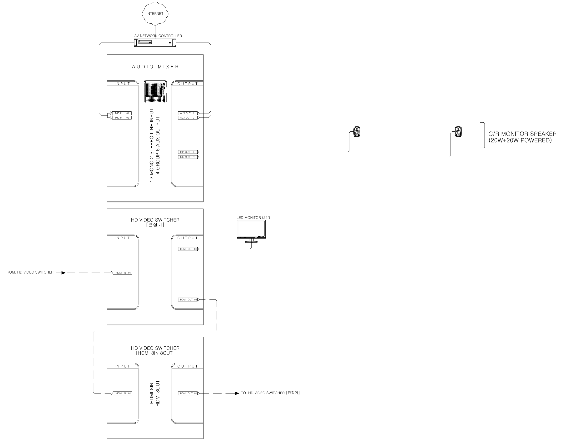
IBS5250-V01 계통도 SCALE : 1/NONE (A3)
