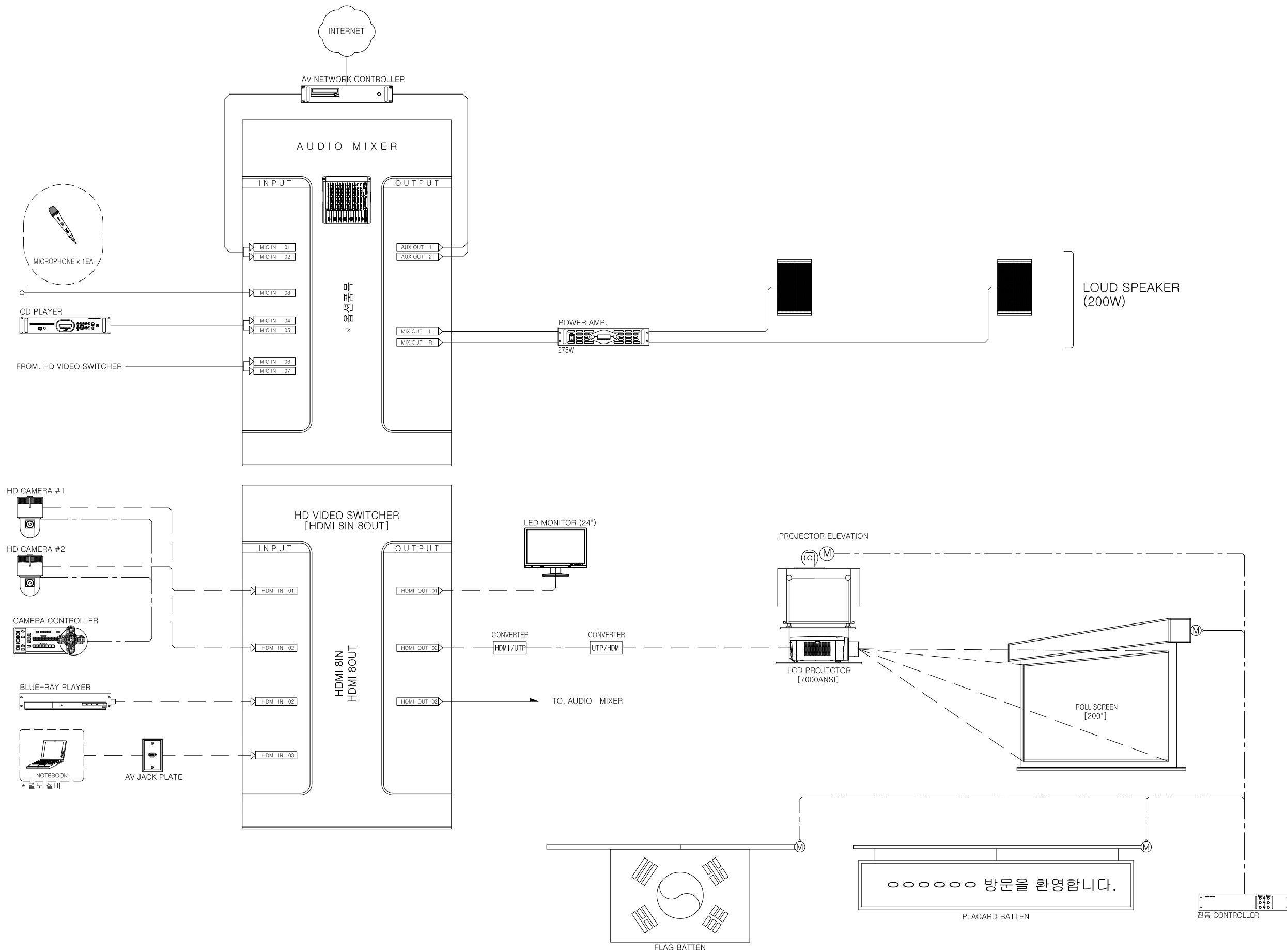
IBS5250-V08A 계통도 SCALE : 1/NONE (A3)
