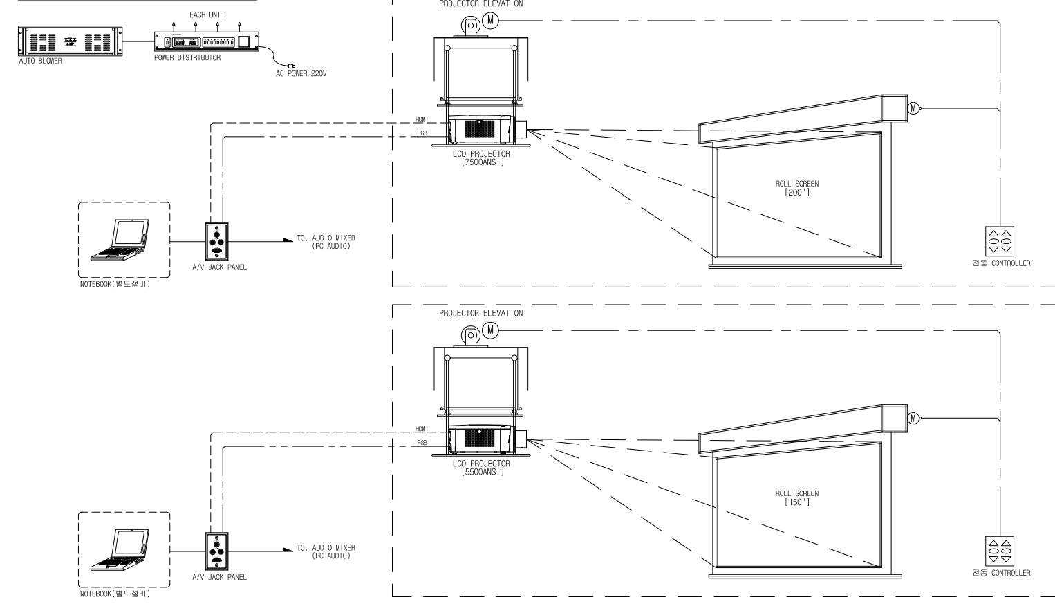
IBS5250-SW30 계통도 SCALE : NONE
